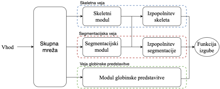
Slika 2: Visokonivojski arhitekturni diagram predlaganega modela SPD. Skupno mrežo ResNet si delijo tri specializirane veje modela, zasnovane za segmentacijo človeškega telesa, napovedovanje skeletnih točk in napoved globinske predstavitve poze.
